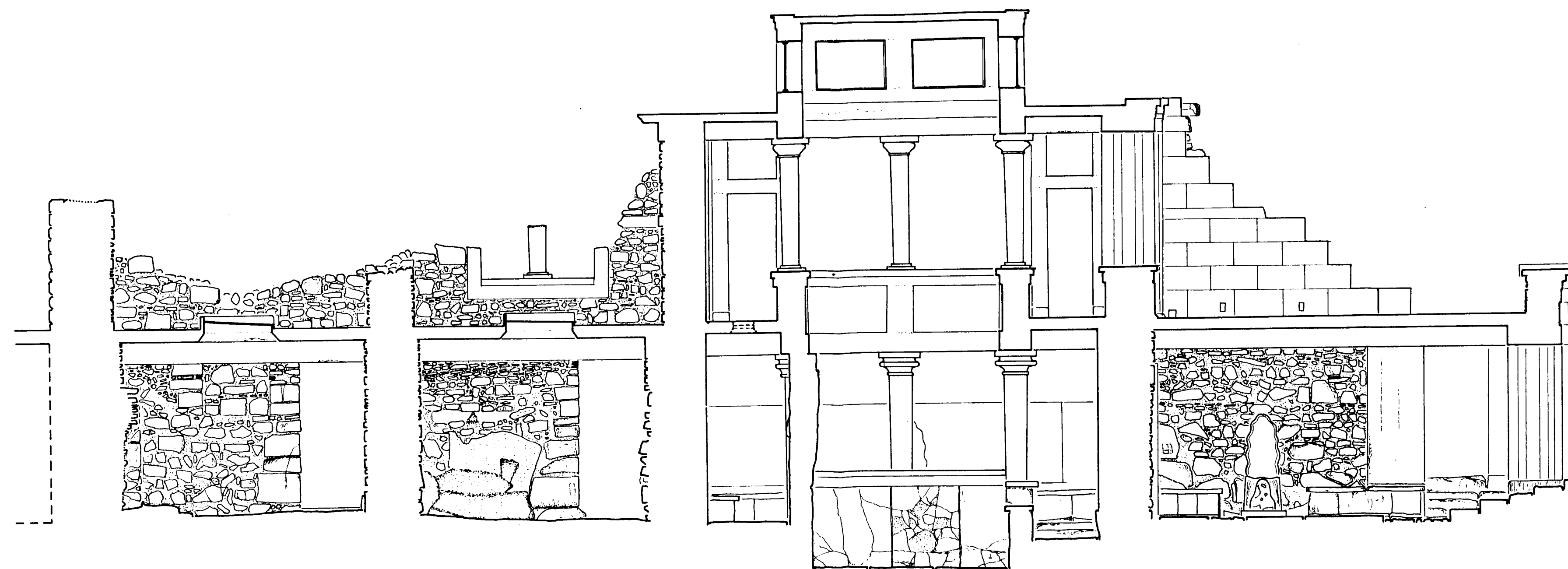
Section A-A
