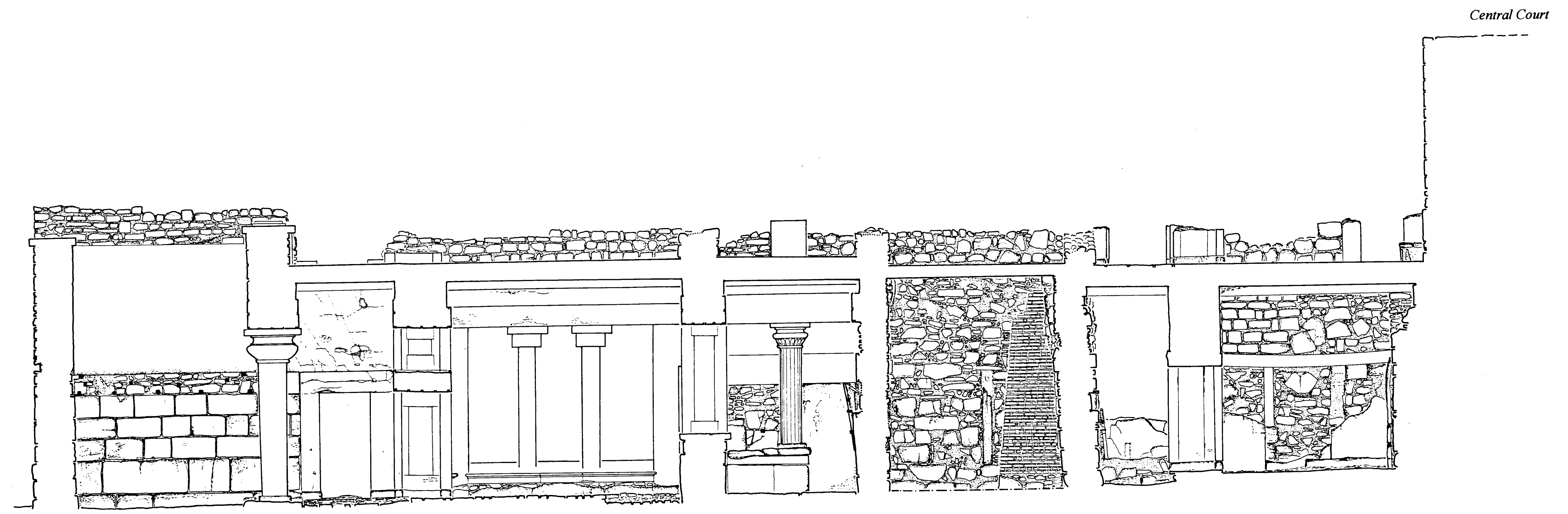
Section A-A
