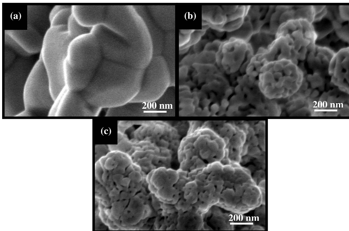
Fig. 2.5 SEM of a) bulk \text{Ta}_2\text{O}_5 ; b) bulk \text{TaON} ; c) bulk \text{Ta}_3\text{N}_5
